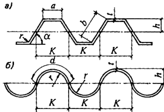
Черт. 12. Расчетная схема сжатого гофрированного листа
