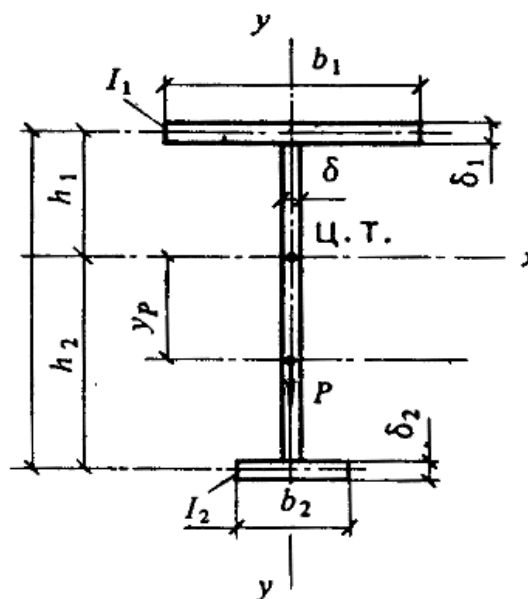
Поперечное сечение балки с развитым верхним поясом
