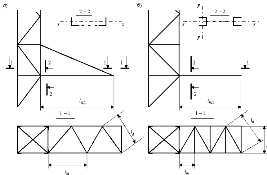
Рис. 21. Схемы траверс а – с треугольной решеткой; б – то же, со стойками
