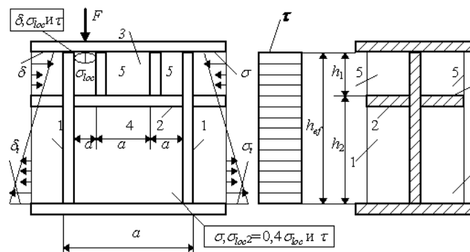
Рис. 14. Схема балки, укрепленной поперечными основными ребрами жесткости (1), продольным ребром жесткости (2), разделяющим отсек стенки на пластинку (3) у сжатого пояса и пластинку (4) у растянутого пояса, а также короткими ребрами жесткости (5)
