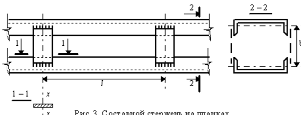
Рис. 3. Составной стержень на планках
