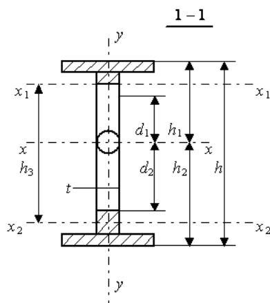
Рис. 23. Схема участка балки с перфорированной стенкой
