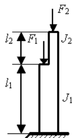
Рис. 24. Схема одноступенчатой колонны
