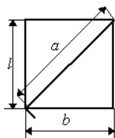
Рис. 2. Схема раскосной решетки
