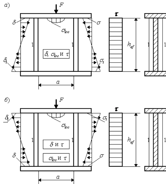
Рис. 12. Схема балки, укрепленной поперечными основными ребрами жесткости (1)
