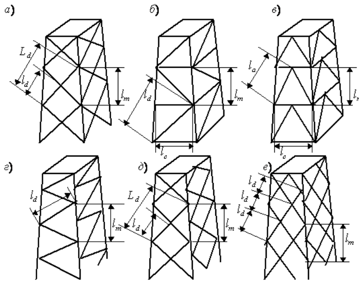
Рис.9*. Схемы пространственных решетчатых конструкций а, б, е – с совмещенными в смежных гранях углами, г, д, е – с несовмещенными в смежных гранях углами
