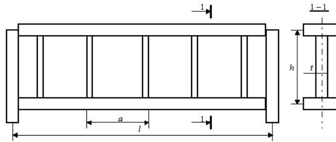
Рис. 22. Схема балки с гибкой стенкой
