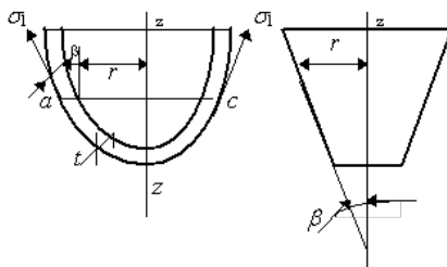
Рис. 17. Схема оболочки вращения
